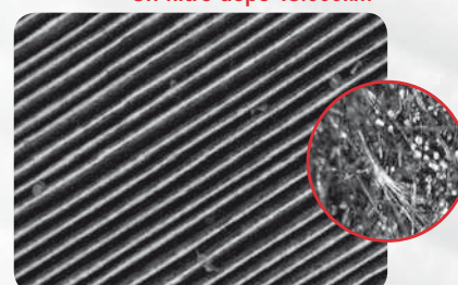
Un filtro dopo 15.000km
