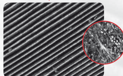
Filtro después de 15 000 km.
